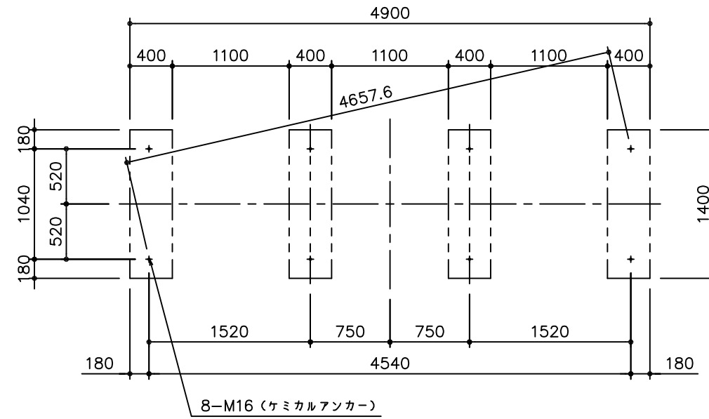
基礎伏図
