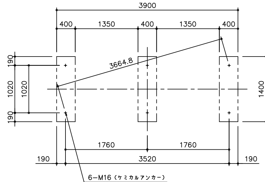
基礎伏図
